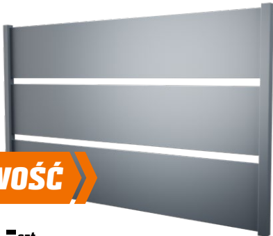
559,- 99 szt. Przęsło ogrodzeniowe Arizona* kolor antracyt mat, wym. 200 x 120 cm, waga 34 kg, np. nr OBI 7020241 Dostępne również: • wym. 200 x 90 cm, waga 26 kg, 569,- szt., nr OBI 7020233 • wym. 200 x 150 cm, waga 41 kg, 799,- szt., nr OBI 7348154
