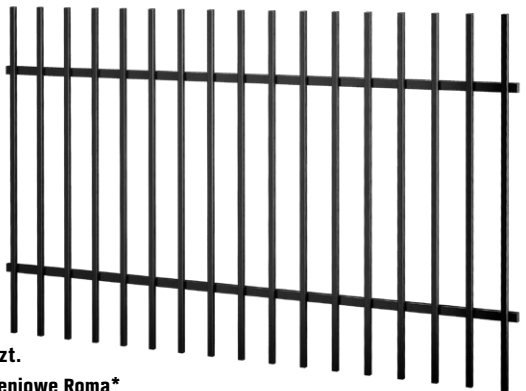
275,- 99 szt. Przęsło ogrodzeniowe Alabama* kolor antracyt, wym. 200 x 120 cm, waga 13,5 kg, nr OBI 7024912 Dostępne również wym. 200 x 150 cm, waga 17 kg, 299,- szt., nr OBI 7024920
