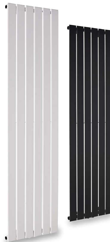
Grzejnik dekoracyjny Vertirad wym. 1800x455 mm, moc 824 W przy temp. 75/65/20°C, kolor biały nr ref. 25113205 nr ref. 25113204 – kolor czarny – 549,00 zł
